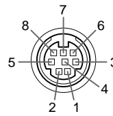
Mini DIN 8 pin connector
