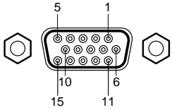
Mini D sub 15 Pin connector
